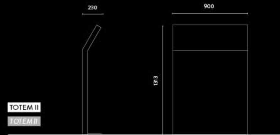
PROFIL PROFILE
